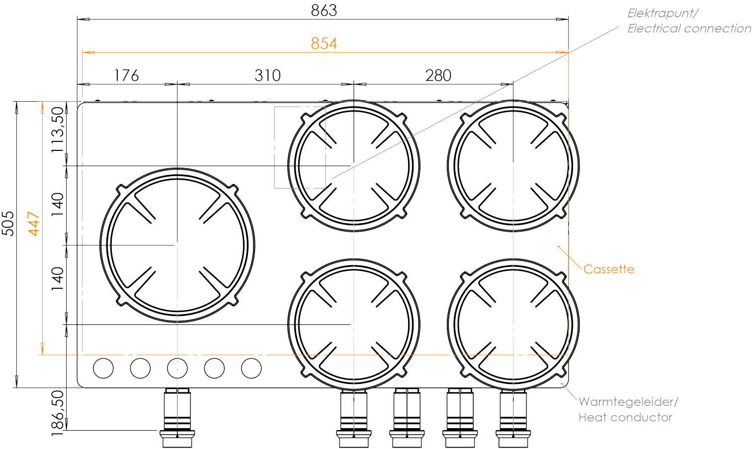
Bovenaanzicht / Top view
