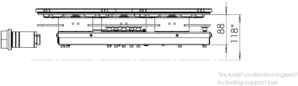
Zijaanzicht / Side view
